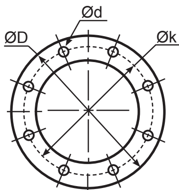
ANSI (ASA) B 16,5
